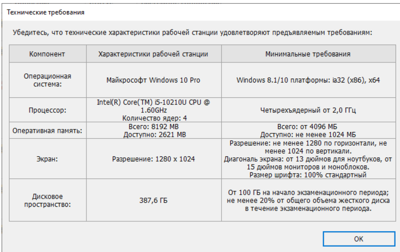
Рис. 6.47. Окно «Технические требования»
